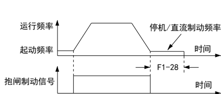
抱闸延迟时序图
