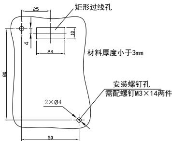
机柜安装操作面板时开孔图
