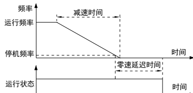
零速延迟时序图
